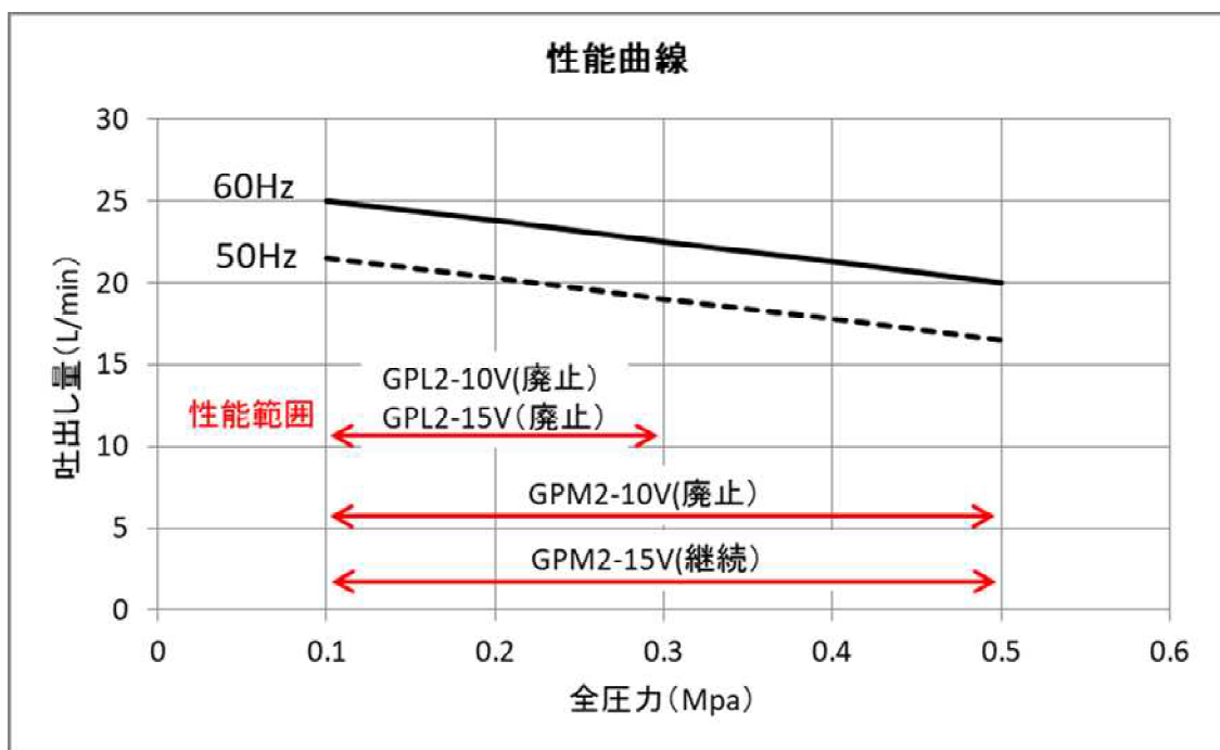
図1. 廃止製品と代替製品の性能曲線
